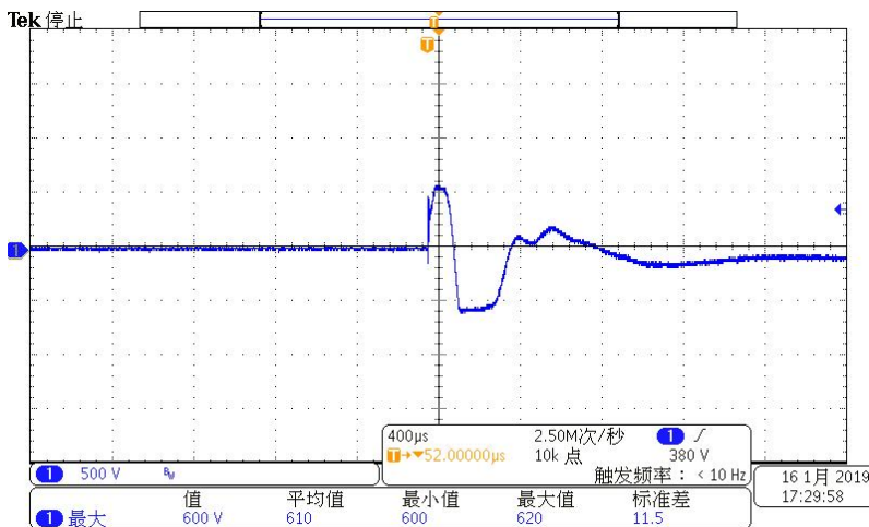
打共模4KV输出端差模残压600V
